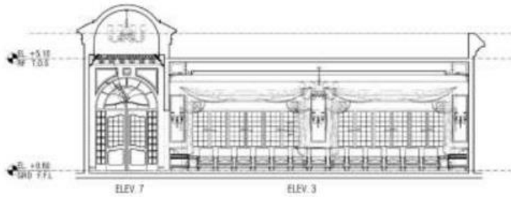
ELEV 7
